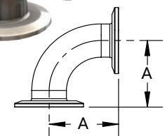
BPE Table DT-4.1.1-3 ASME BPE 2019
