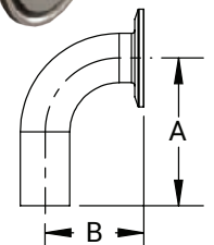
BPE Table DT-4.1.1-2 ASME BPE 2019
